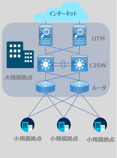
従来のオンプレミス型UTM構成
